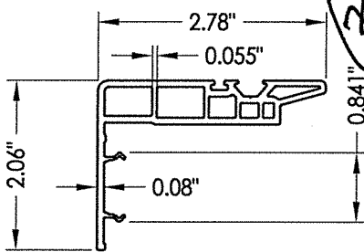
5 INTERLOCK 8573-356-D63
