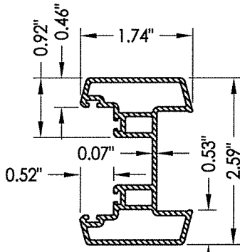
40 ASTRAGAL 356-A60
